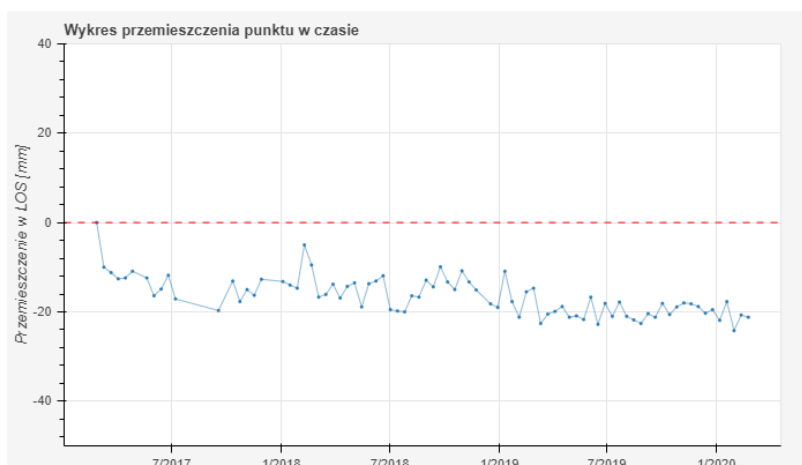
Fig. 7 Point ID 88405 - displacement in LOS values (descending dataset)
