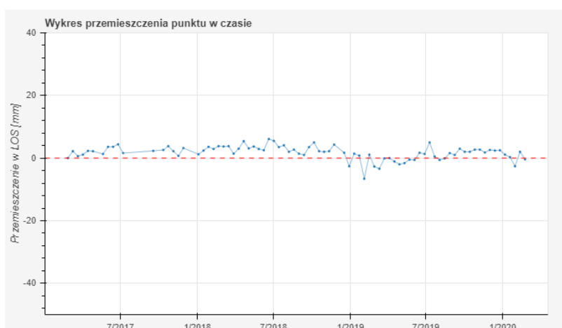
Fig. 8 Point ID 89464 - displacement in LOS values (descending dataset)
